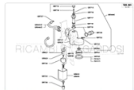
GRUPPO ELETTROVALVOLA - Tav.001
