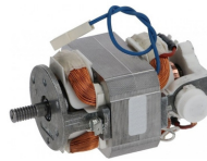
RG254426 Motore a cinghia macinados. 230V 60Hz Grinder motor belt-driven 230V 60Hz
